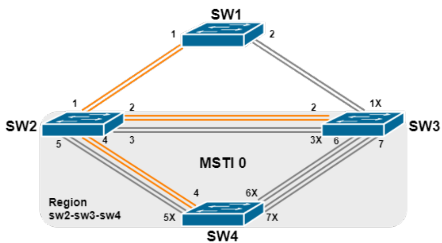
Рис. 13: Топология MSTI 0
