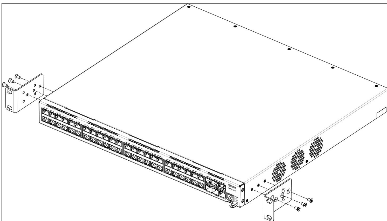
Рисунок 2 – Крепление кронштейнов к коммутатору
