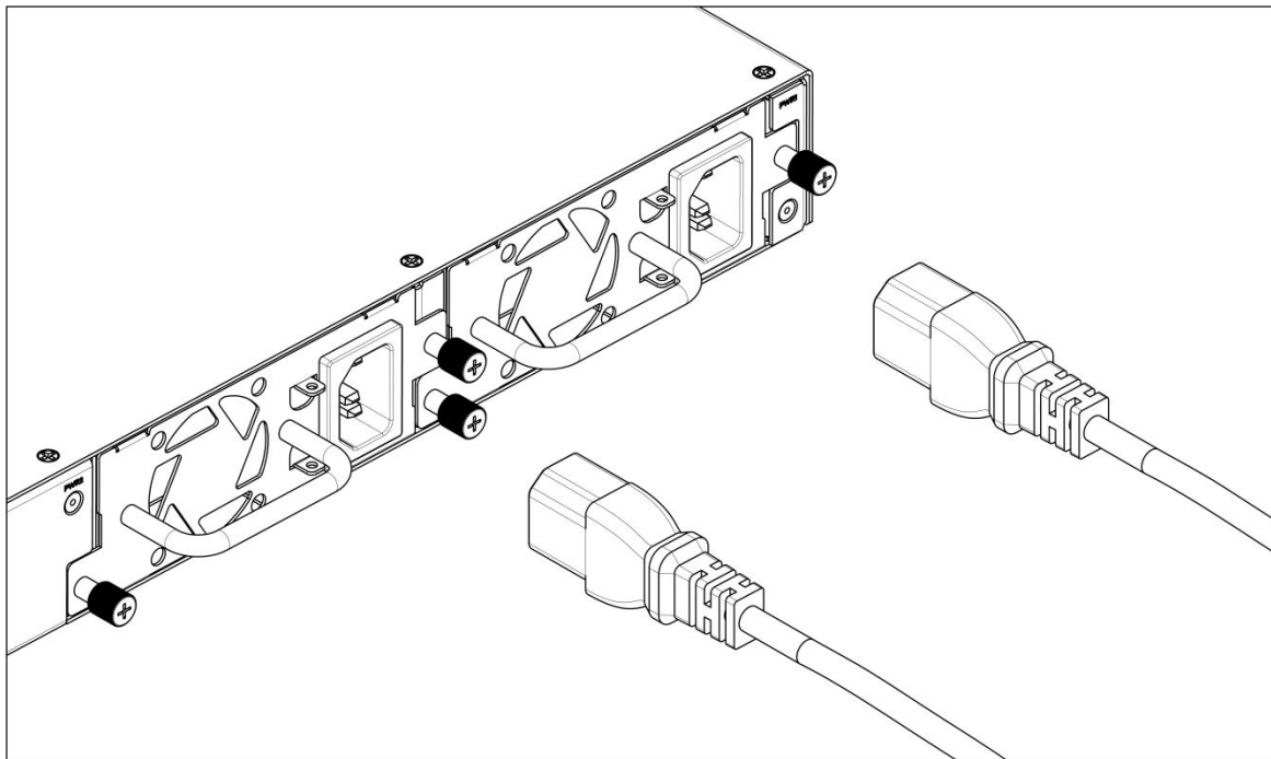
Рисунок 4 – Подключение кабеля питания
