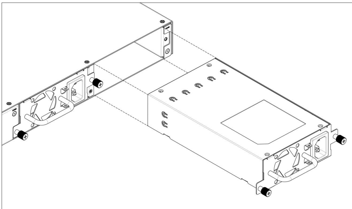
Рисунок 5 – Замена блока питания
