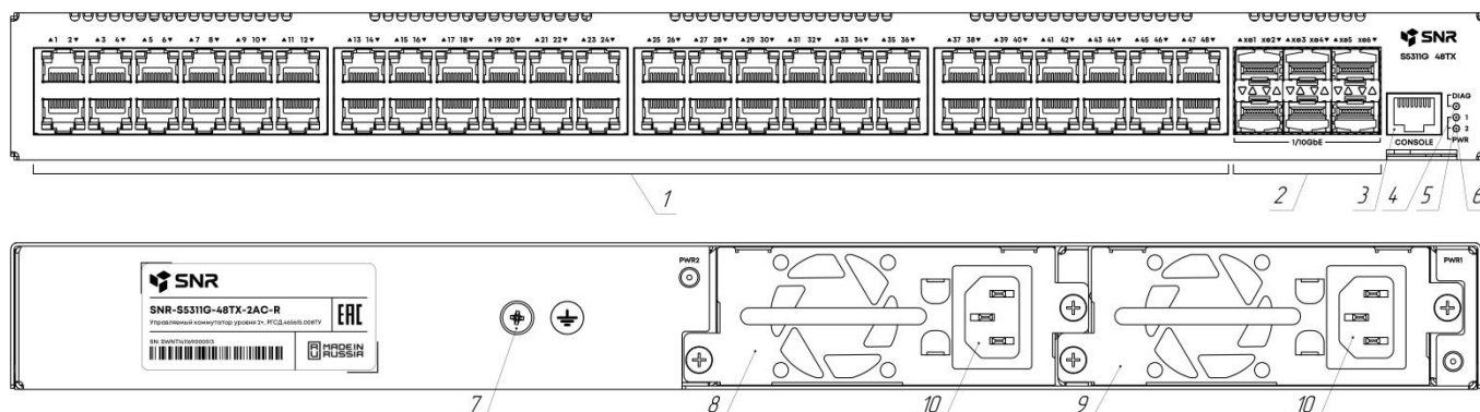
Рисунок 1 – Разъёмы, индикаторы и органы управления коммутатора
